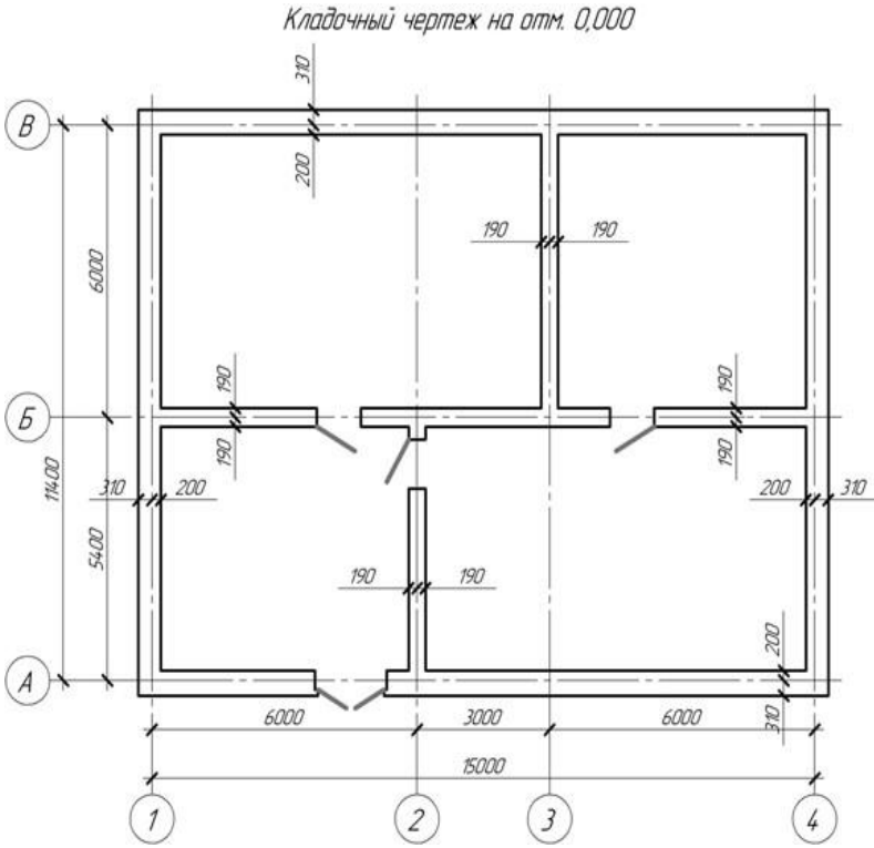
Рисунок 1. Кладочный чертеж к заданию 1 Модуля 2
